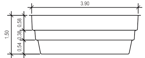
Vue de Coupe/Querschnitt/Sección 1
