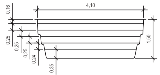
Vue de Coupe/Querschnitt/Sección 3
