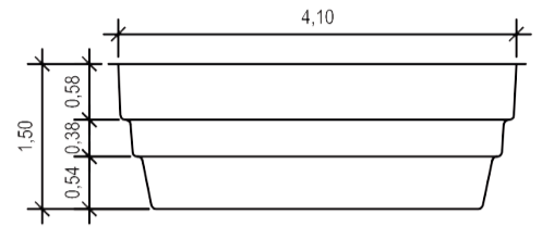
Vue de Coupe/Querschnitt/Sección 1
