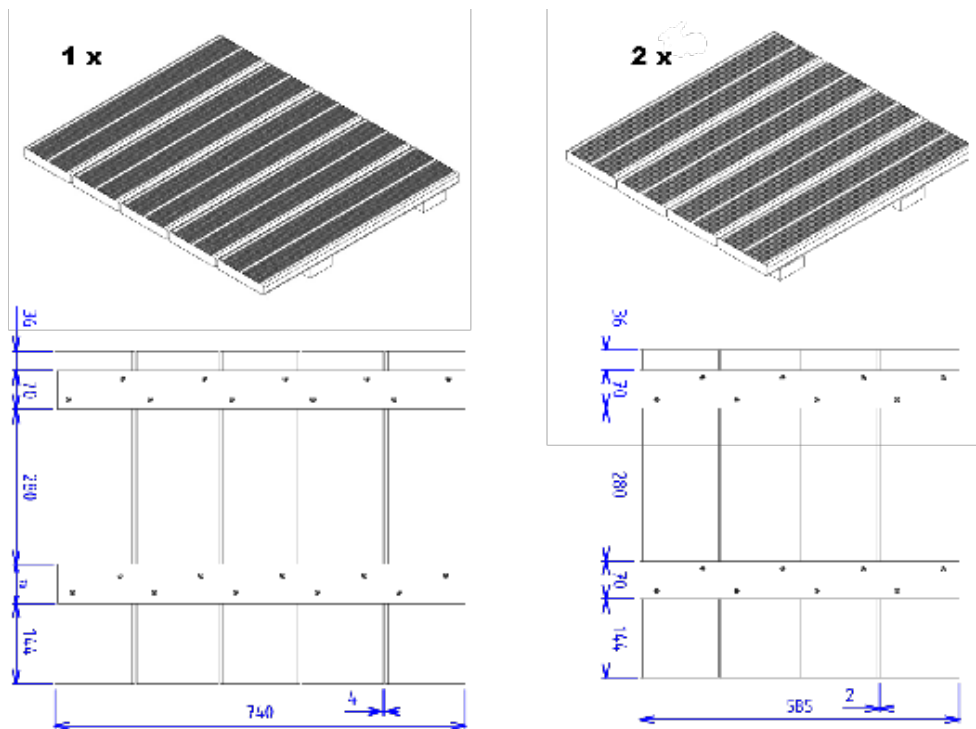
Abbildung 51 – Montage der Holzroste
